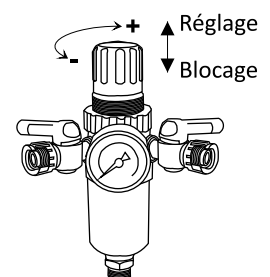
Epurateur-détendeur
