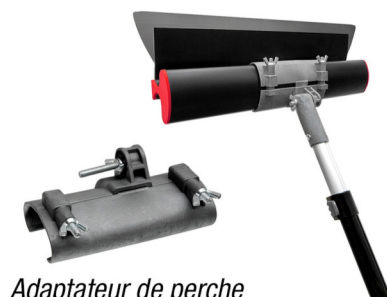
Perche télescopique réf. 44 16 52
