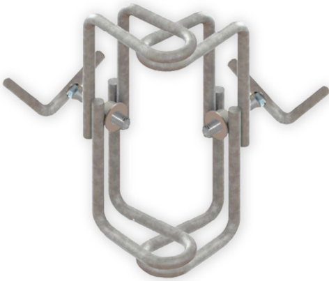
Coulisseau d'angle fil acier galvanisé diam. 12 mm, 2 manettes de serrage.
