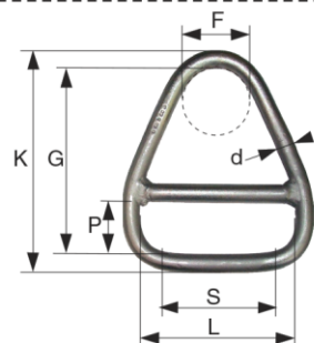
ANNEAU FEMELLE ref. 5072
