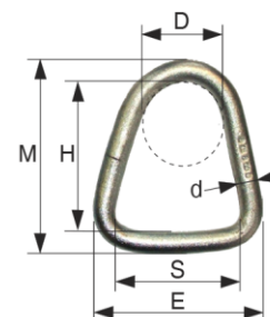
ANNEAU MÂLE ref. 5070
