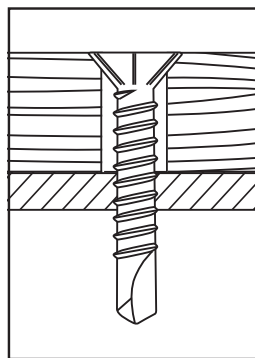
3 Formation du taraudage par déformation.
