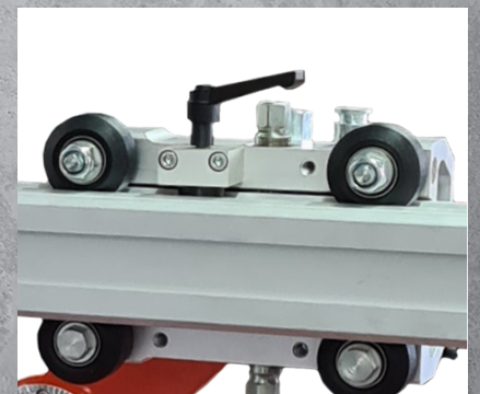
Guidage par roulements
