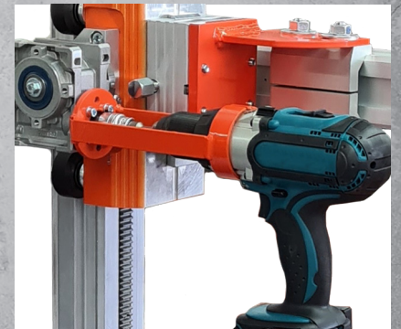
Avance par batterie avec engrenage à vis sans fin
