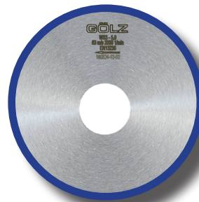
Alésage 60,0 (Autres alésages et perçages spécial sur demande)
