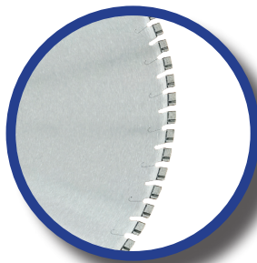
Segments spécifique avec encoche, soudés laser
