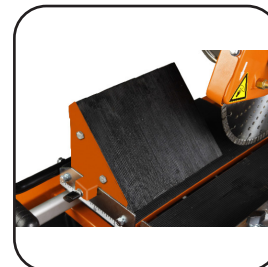
Coupe biseau 45°
